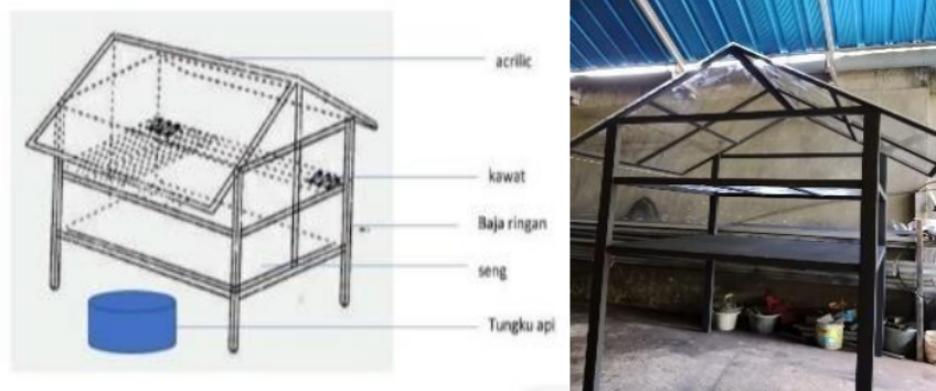
Gambar 2, Desain alat pengering hybrid dan alat pengeringan hybrid (Bidayani, et al, 2022)
