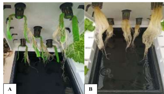
Gambar 1. Perakaran tanaman : a) sistim wick, b) sistim kratky, umur tanaman 18 Hari Setelah Tanam (35 Hari Setelah Semai benih).
