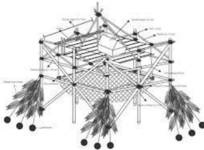
Gambar 2. Ilustrasi Rekayasa Rumpon Pada Bagan Tancap
