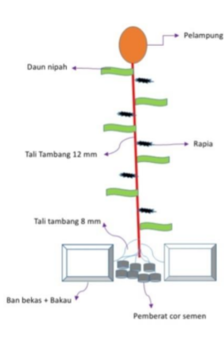
Gambar 3. Desain Rumpon Portable (Sumber: Ardiansyah, 2021)
