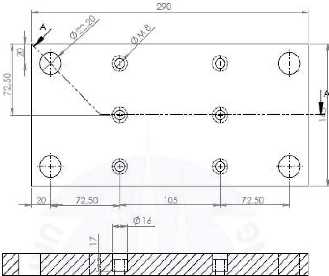
SECTION A-A SCALE 1 : 2
