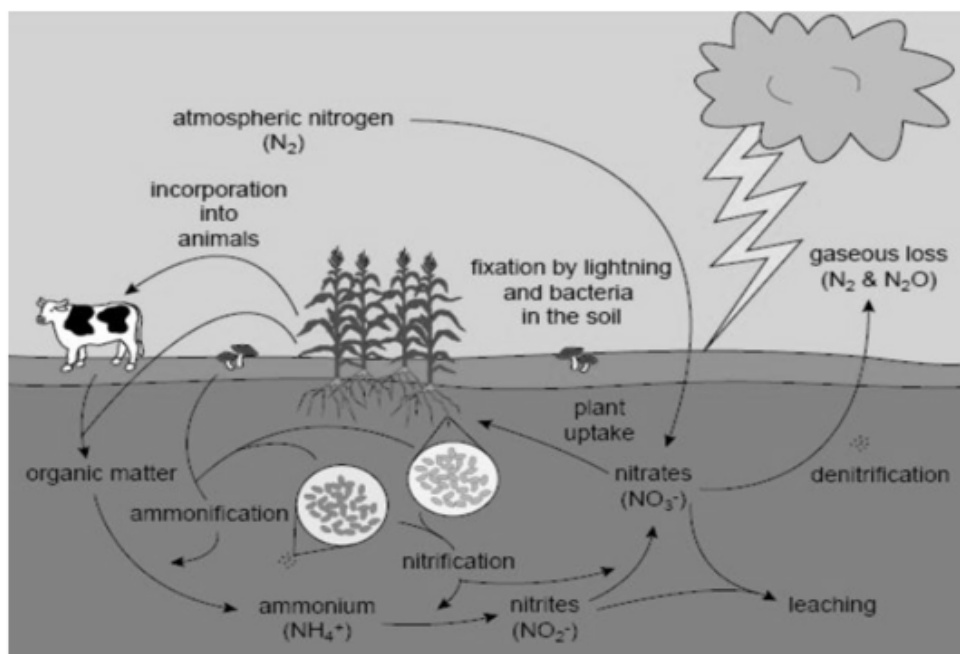
Gambar 5. Ilustrasi siklus nitrogen yang terjadi di biosfer [22] .
