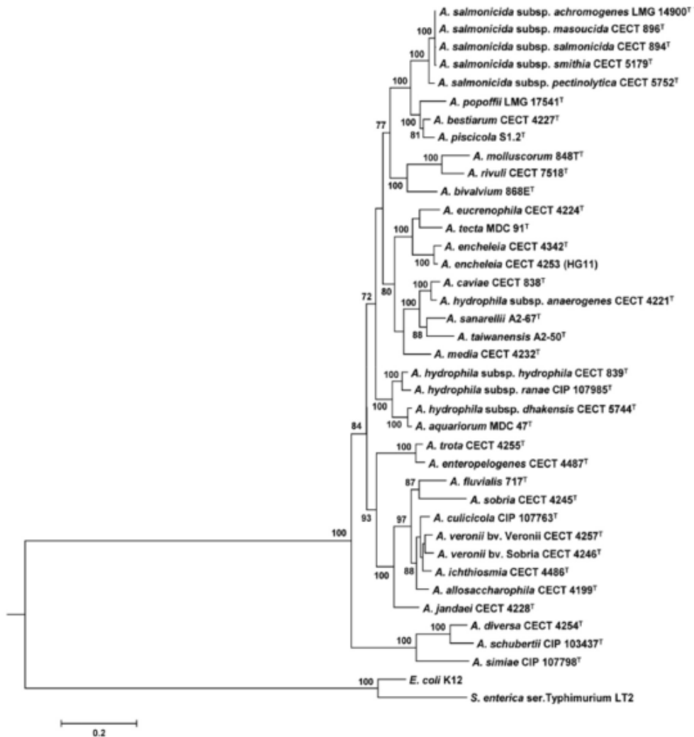
Gambar 45. Pohon filogenetik bakteri Aeromonas [109] .
