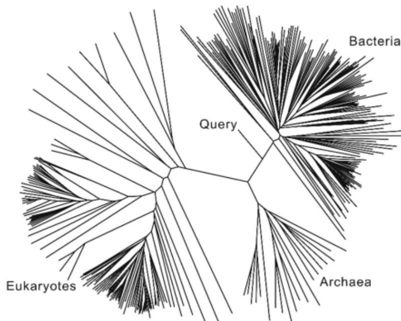
Gambar 7. Filogenetik domain organisme: Eukariot, Bakteria, dan Archaea [29] .
