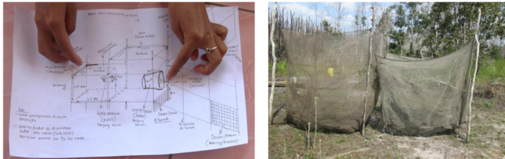
Gambar 3. Desain gambar sero (kiri) dan bentuk alat tangkap sero (kanan) yang dibuat masyarakat.
