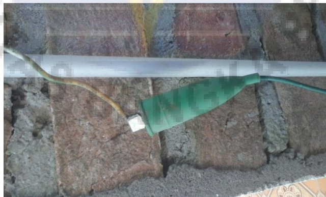
Pemasangan Kabel Penghubung ke Pentanahan Pada kWh Meter
