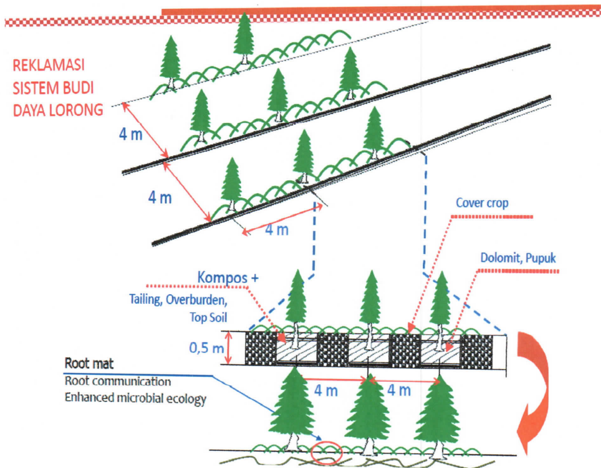
Gambar 20 Ilustrasi disain teknis reklamasi (Inonu 2010)
