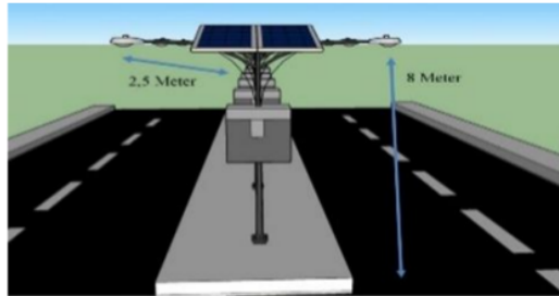
Gambar 6. Ukuran Ketinggian Tiang dan Stang Ornamen PJU
