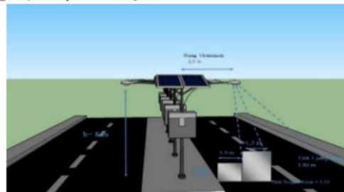
Gambar 7. Pengukuran Lampu PJU
